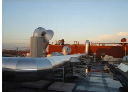
Abb. 27: Drei-Kammer-Wärmetauscher mit Abluftführung über Dach
