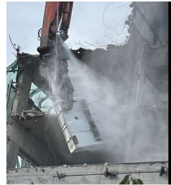
Staubbindung am eingesetzten Longfront-Bagger
